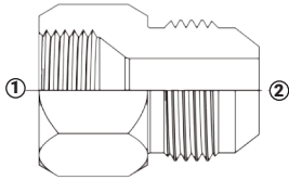
(1) Hembra JIC 37° (2) Macho JIC 37°
