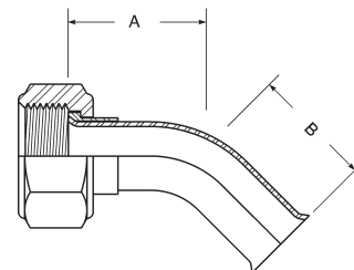
Rosca Hembra SAE 37° (JIC) x Extremo Soldable
