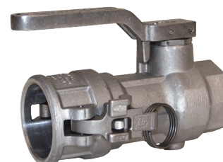
Acople x 3" hembra NPT
