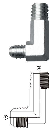
(1) Macho JIC 37° (2) Macho NPTF SAE 071502
