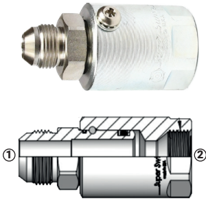
(1) Macho JIC 37° (2) Hembra JIC 37°
