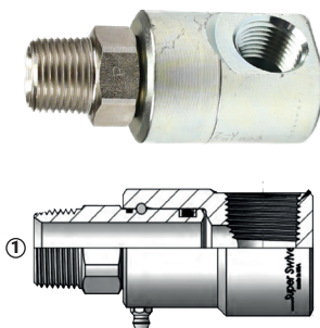
(1) Macho NPTF (2) Hembra NPTF
