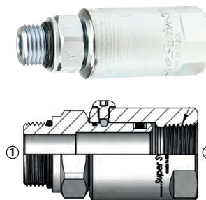
(1) Macho ORB (2) Hembra NPTF
